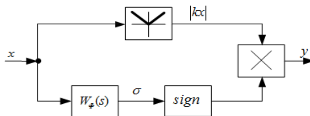
1 – блок определения модуля; 2 – интегро-дифференцирующее звено; 3 – знаковый оператор Sign, 4 – устройство перемножения
