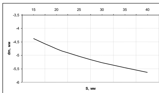
Рисунок 5 – Зависимость абсолютной погрешности измерения уровня от расстояния сенсора до вертикальной электропроводной цилиндрической стенки
