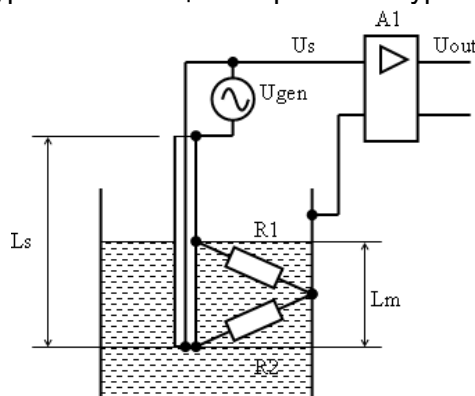
Рисунок 1 – Функциональная схема измерения уровня потенциометрическим уровнемером
